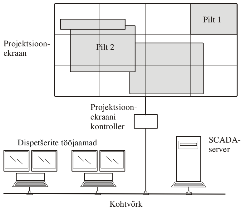
Joonis 5.3 Projektsioonekraani lülitusskeem
