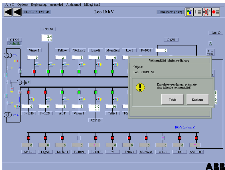
Joonis 5.11 Alajaama skeem ja lülitamise dialoogiaknad
