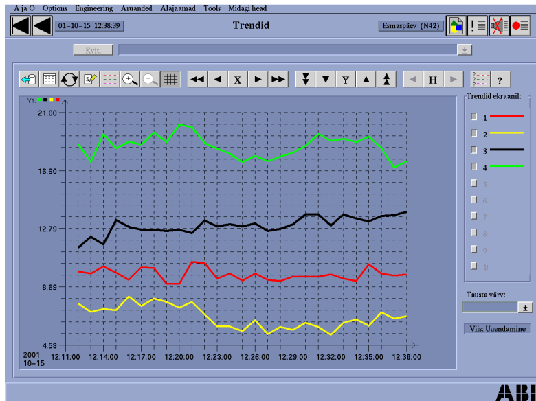
Joonis 5.8 Mõõtmiste trendipilt
