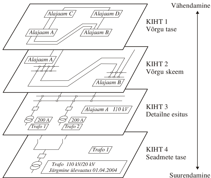
Joonis 5.4 Elektrivõrgu skeemi kihid
