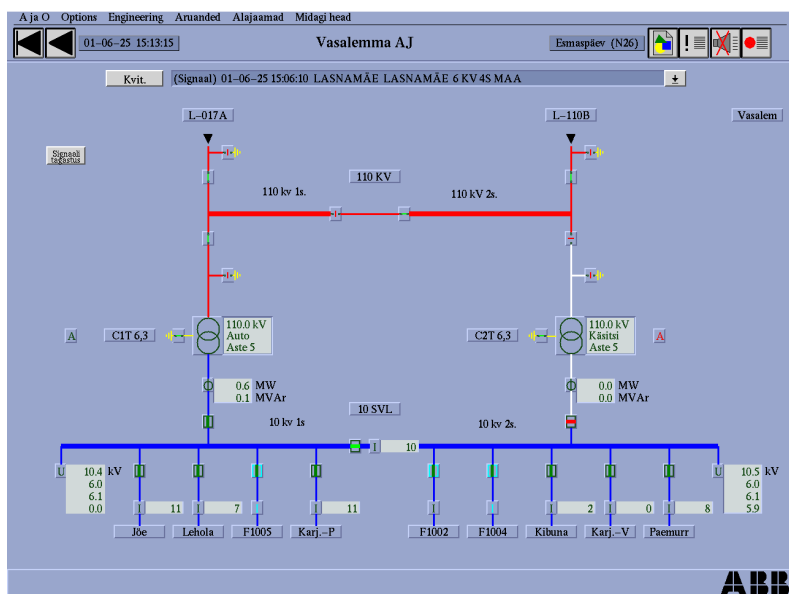
Joonis 5.6 Alajaama skeem
