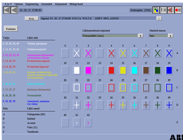
Joonis 5.14 Võimsuslülitid kujundi šabloonid
